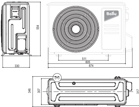
Размеры внешних блоков BM2OI-FM/out-14HN8_V1/EU, BM2OI-FM/out-18HN8_V1/EU:
